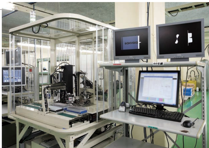
長岡工場極小径専用再研磨ライン ADP repointing line, Nagaoka factory
